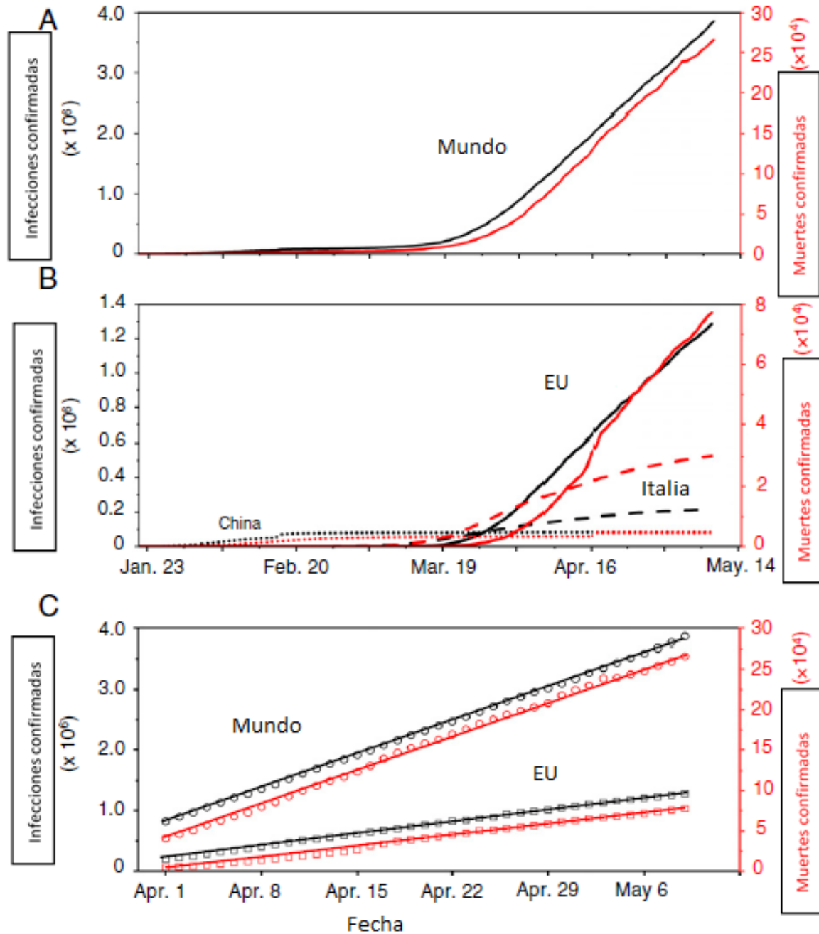
Fig. 1. Distintas tendencias globales de la pandemia COVID-19. (A) Infecciones y muertes totales confirmadas en todo el mundo. (B) Comparación de las infecciones confirmadas y de los fallecimientos en China, Italia y en Estados Unidos. (C) Regresión lineal de los casos confirmados de infecciones y fallecimientos globales y en los Estados Unidos del 1ro de abril al 9 de mayo, 2020; la regresión lineal es, respectivamente y = 79,398x + 810,167 ( R^2 = 0.999 ) para infecciones y y = 6,075x + 39,409 ( R^2 = 0.998 ) para fallecimientos globales, y y = 28,971x + 201,187 ( R^2 = 0.999 ) para infecciones y y = 2,059x + 243 ( R^2 = 0.995 ) para fallecimientos en los Estados Unidos. El eje izquierdo y el color negro corresponden al número de infecciones confirmadas, y el eje derecho y el color rojo corresponden a los fallecimientos confirmados.
